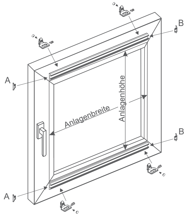
Montage verspannt auf dem Rahmen
