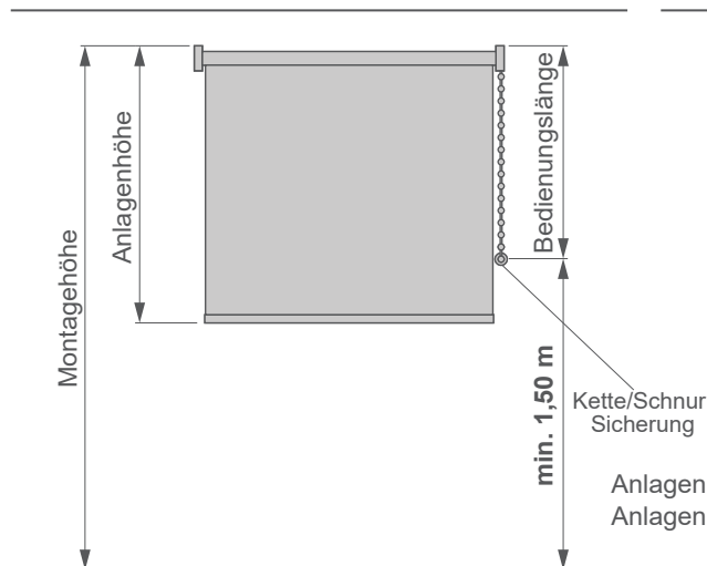
Montagehöhe bekannt
