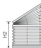
Gespannte Slopeanlage mit Bediengriff und Spannschiene.
