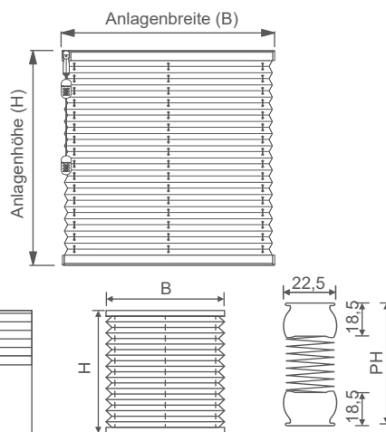
Freihängende Anlage mit Schnurzugbedienung.
