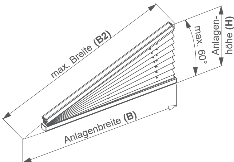
Feststehende Dreieckanlage.
