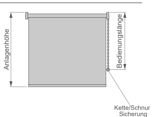
Montagehöhe unbekannt
