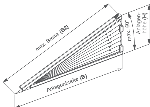
Freihängende Dreieckanlage mit Schnurzugbedienung.
