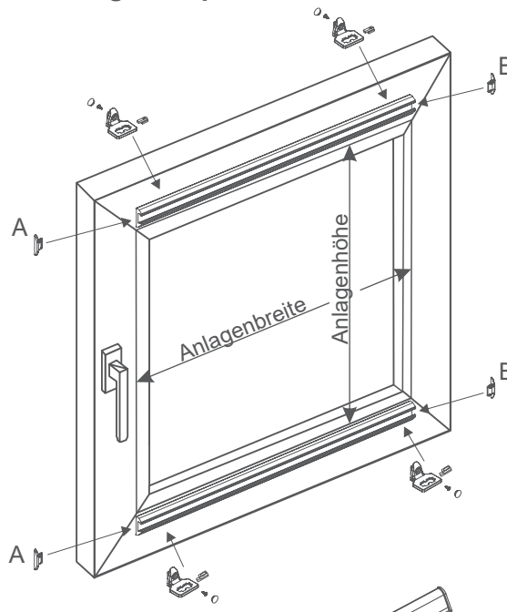
Montage verspannt auf dem Rahmen
