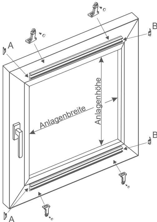
Montage verspannt im Falz
