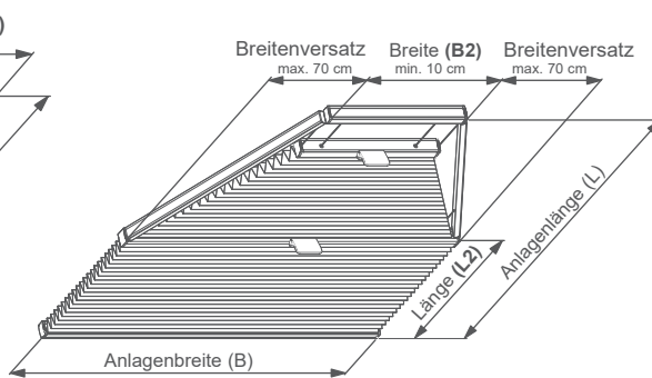
Gespannte 6-Eckanlage mit Drahtspannung und Bediengriff.
