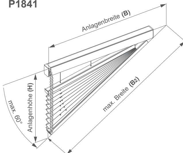
Gespannte Dreieckanlage mit Kettenzugbedienung
