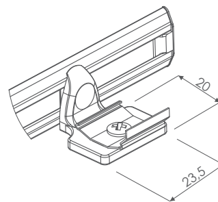
Clip-Befestigung Farben: weiß, silber
