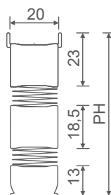
Gespannte 6-Eckanlage mit Bediengriff und Spannschiene.
