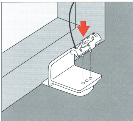
Cosiflor F mit Pendelsicherung Cosiflor F with guide wire Cosiflor F koordrem en koordgeleiding Cosiflor F avec immobilisation Cosiflor F с фиксацией откачения
